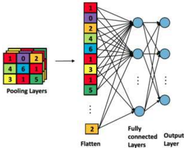
Figura 9 - Exemplo de Flatten com Fully connected.
